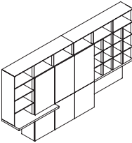
ED98 W3830•D560•H2130(mm)
