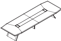
ED78 W4800•D1600•H760(mm)
